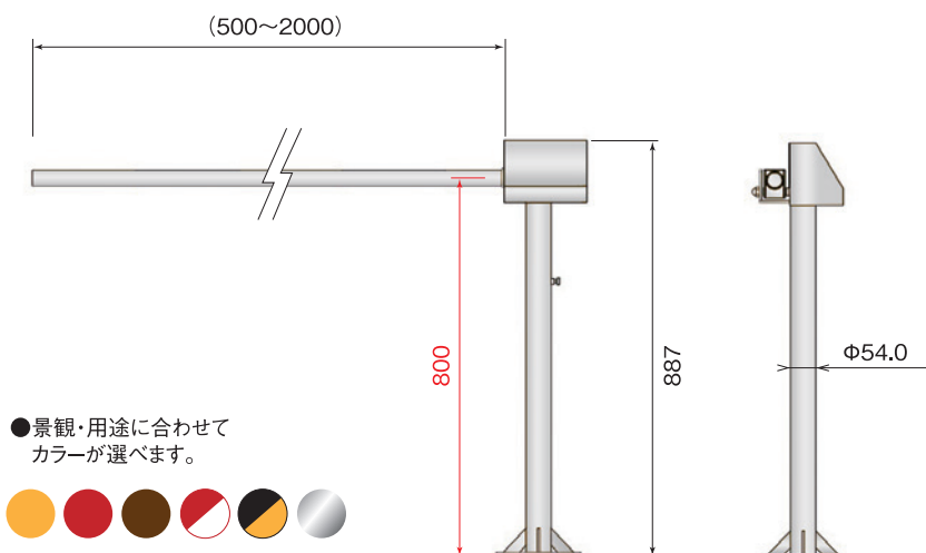
正面図
